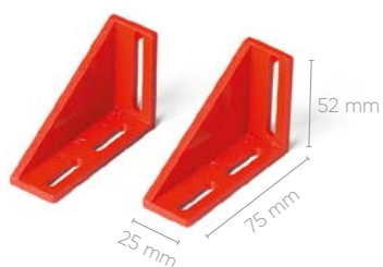
PAIRE DE SUPPORTS PRISMATIQUES
