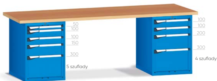
Szafa wym. 561x726x800 h (27x36 Eh) mm
