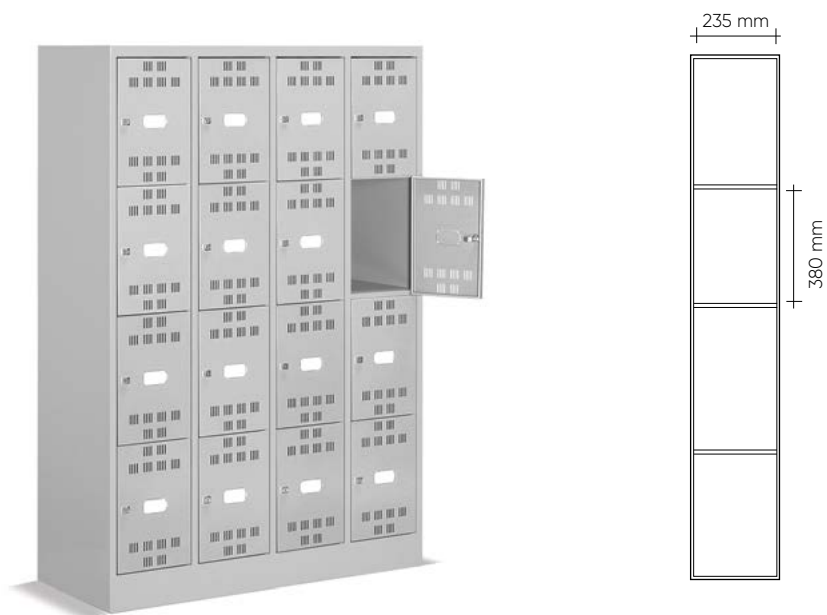
Beispiel mit 16 Abteilen
