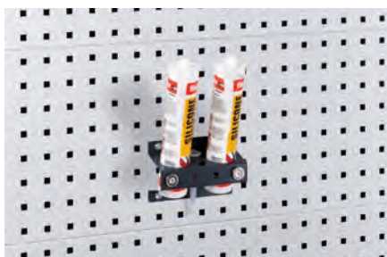
Abgewinkelter Silikonkartuschenhalter mit 2 Stellen
